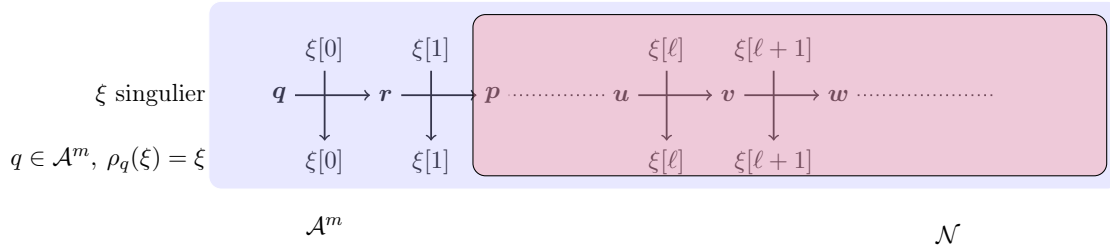
FIGURE III.1 – Si \xi est singulier, alors un de ses suffixe est stabilisé par un élément du noyau.
