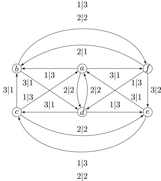
FIGURE I.11 – Un automate à 3 lettres 6 états inversible réversible non-biréversible.
