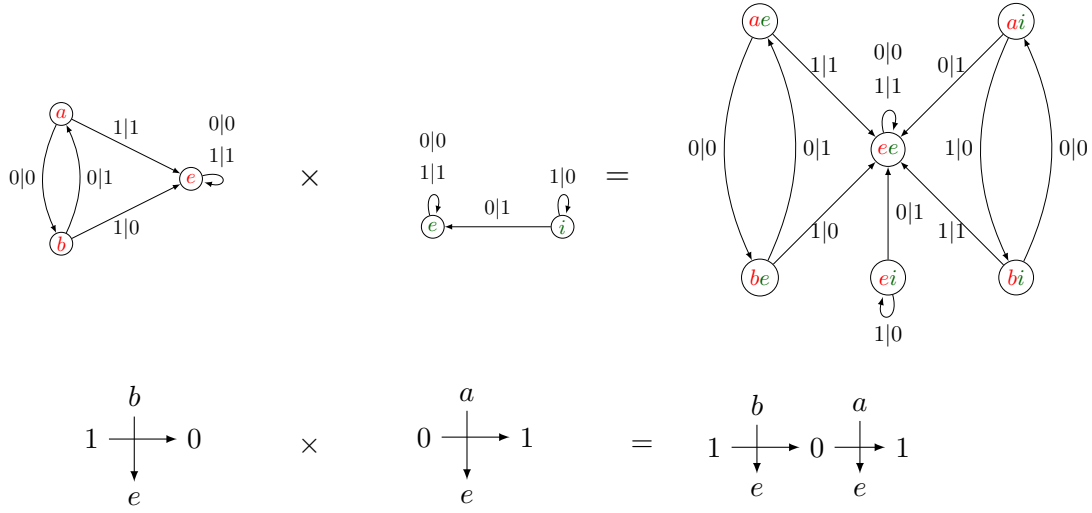
FIGURE I.17 – Produit de l'automate de la Basilique avec la machine à additionner.
