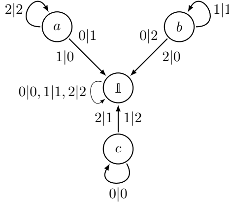
FIGURE III.3 – L'automate (contractant) engendrant le groupe des tours de Hanoï H^{(3)} .
