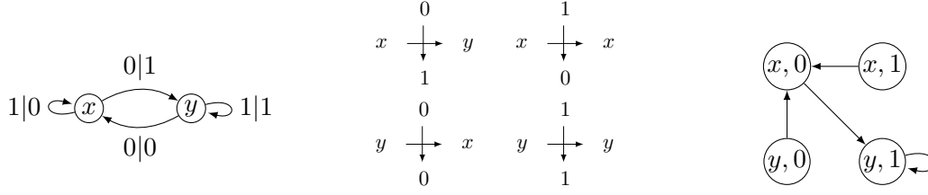
FIGURE I.8 – L'automate de Mealy \mathcal{L} engendrant le groupe de l'allumeur de réverbères, son ensemble de transitions en croix, et son graphe en hélice \mathcal{H}_{1,1}(\mathcal{L}) .
