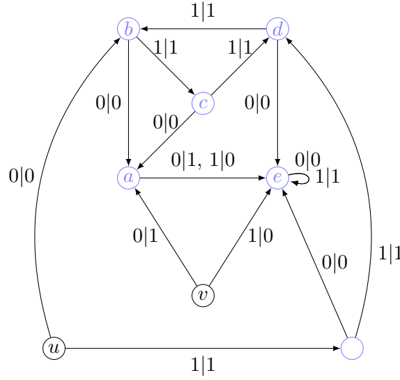
FIGURE I.22 – L'automate d'Alešin. Le groupe \langle u, v \rangle est un groupe infini de Burnside.
