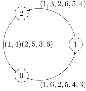
FIGURE IV.4 – Un automate cyclique à 6 lettres et 3 états, engendrant (A_6 \times A_6 \times A_6) \rtimes \langle (1, \pi, \pi) \rangle_c .
