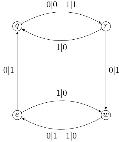
FIGURE II.13 – Automate \mathcal{H} ayant un élément d'ordre infini [27, 68].
