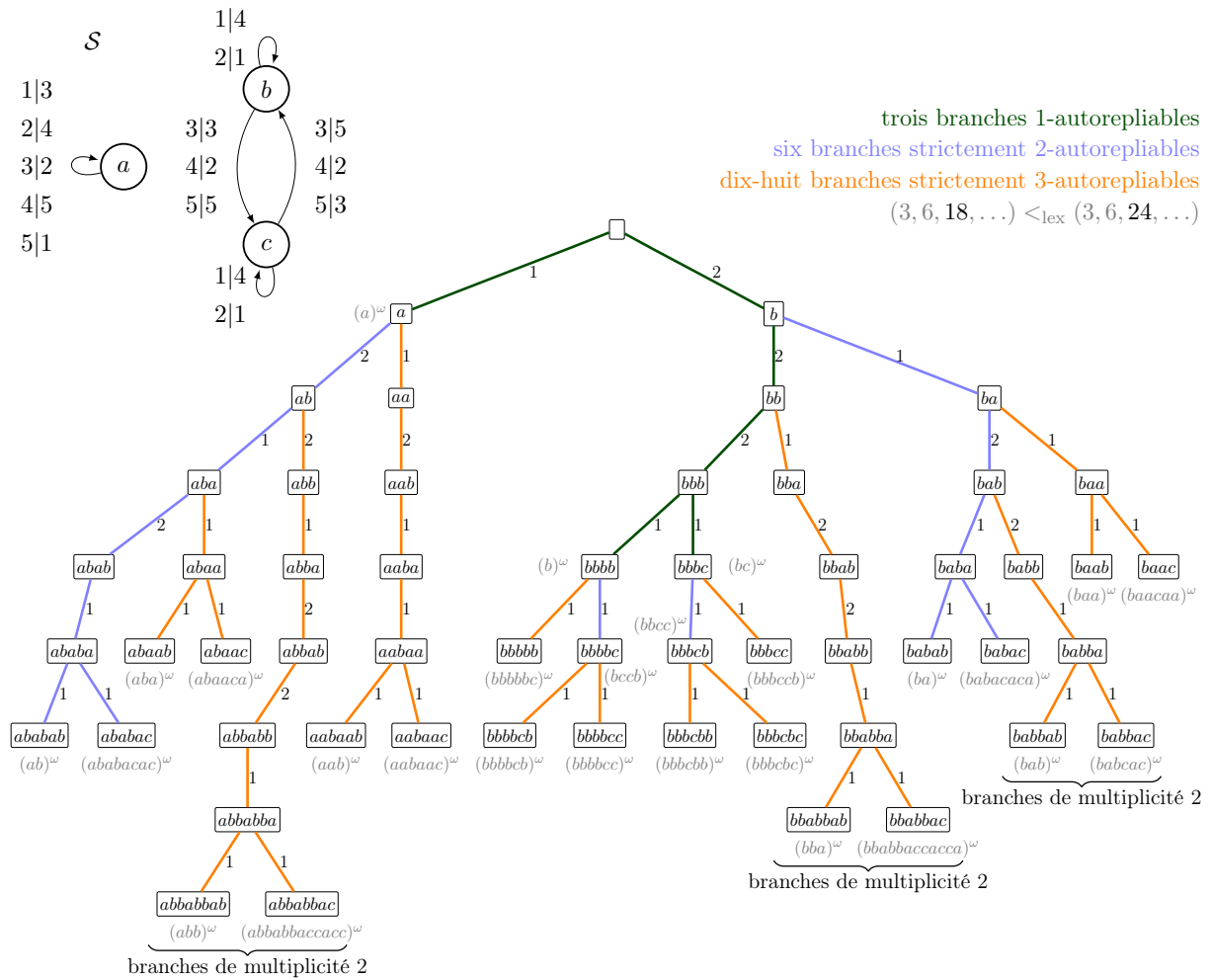
FIGURE II.14 – Dénombrement des chemins strictement auto-repliants d'un automate \mathcal{S} .
