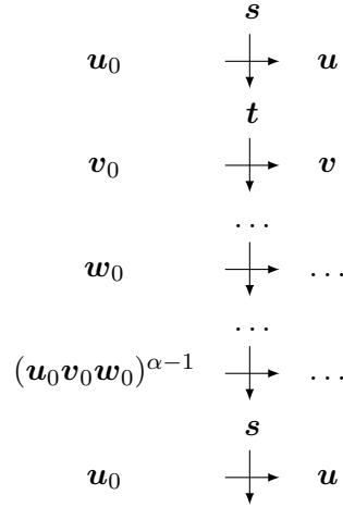
FIGURE II.8 – Extension de la propriété ( Ubiquité ) à n'importe quelle tige.
