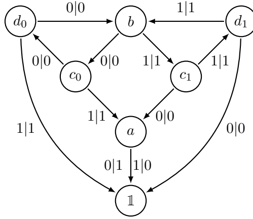
FIGURE III.5 – Une version déformée de l'automate de Grigorchuk ayant un nombre indénombrable de points singuliers. Ce groupe est fractal et contactant et vérifie (000 + 111)^\omega \subset \kappa .
