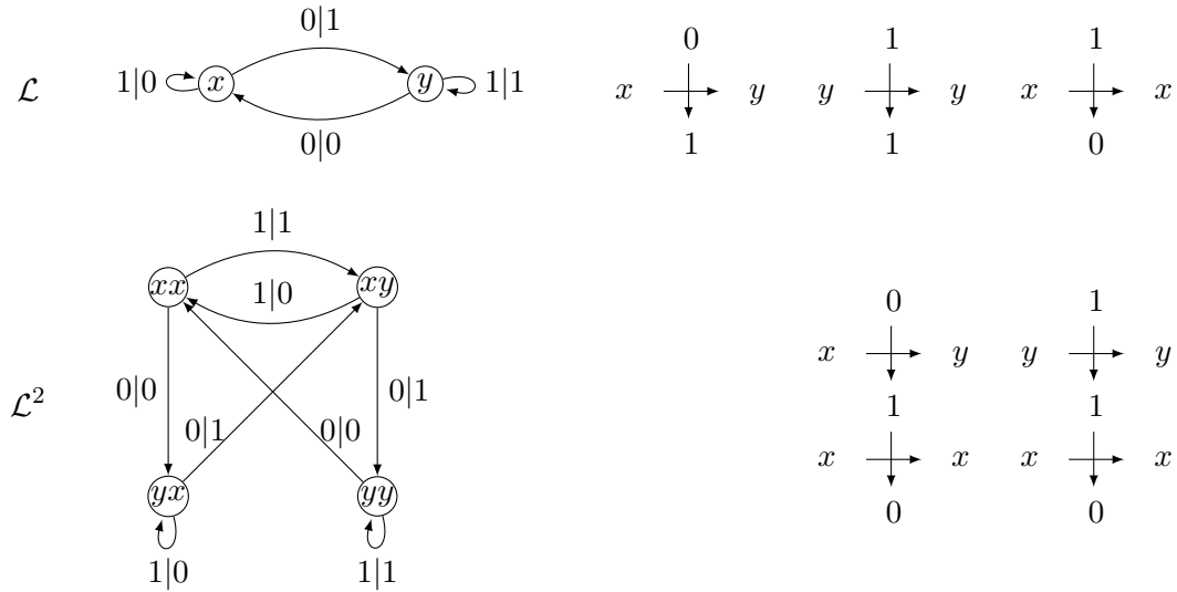
FIGURE II.3 – Un automate de l'allumeur de réverbères \mathcal{L} inversible, réversible et non-corréversible et son carré, qui n'est pas non plus corréversible.
