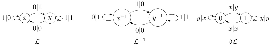
FIGURE I.9 – L'automate \mathcal{L} de l'allumeur de réverbères, son inverse \mathcal{L}^{-1} , et son dual \mathfrak{d}\mathcal{L} .
