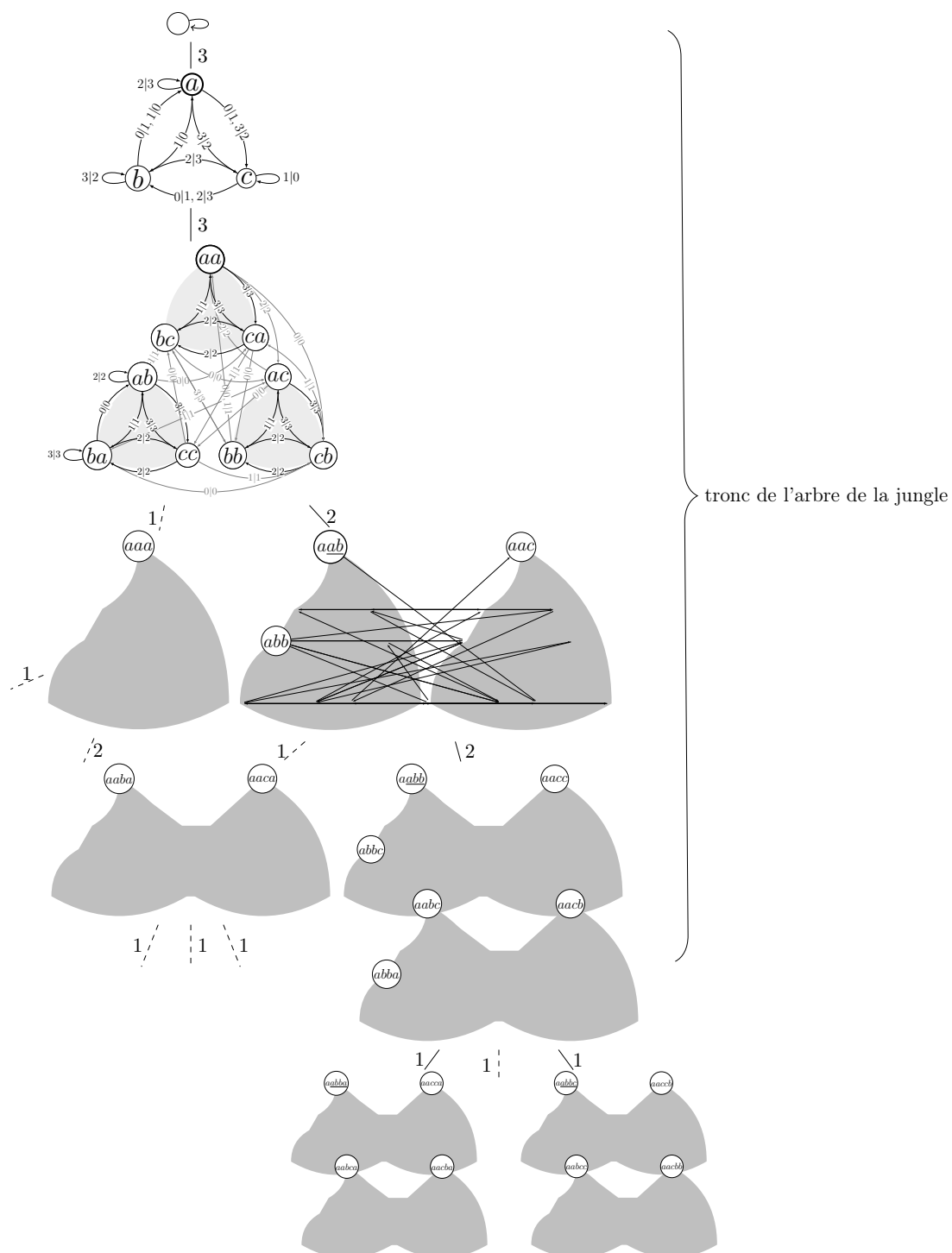
FIGURE II.7 – Un exemple des premiers niveaux de l'arbre de Schreier (tous les sommets et arêtes) dont on extrait un arbre de la jungle (arêtes pleines). Ici \lambda = 4 et l'arité vaut 2.
