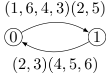
FIGURE IV.3 – Un automate cyclique à 6 lettres et 2 états, engendrant S_6^2 .
