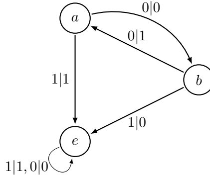
FIGURE I.16 – L'automate engendrant le groupe de la Basilique.
