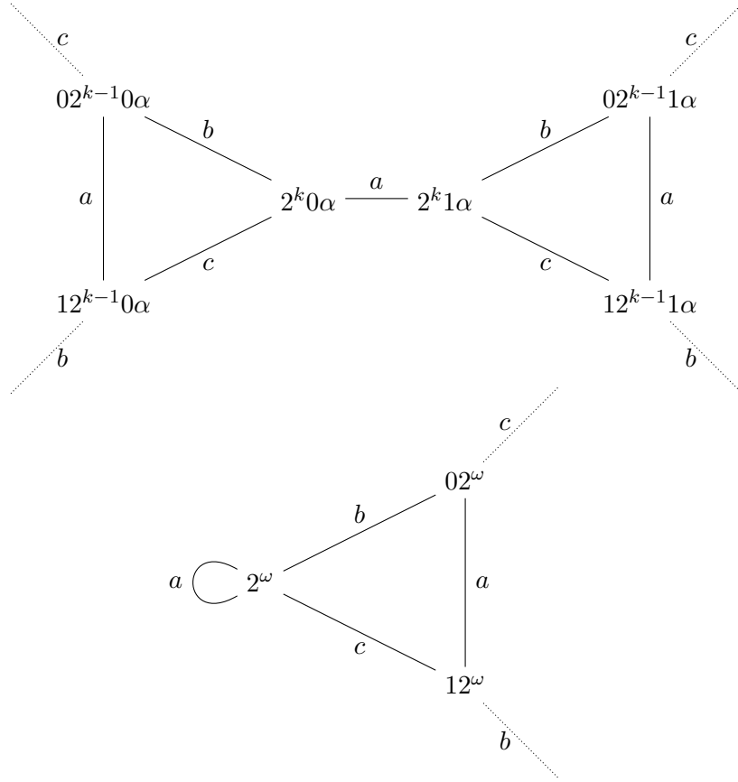
FIGURE III.8 – Une partie d'un graphe de Schreier (infini) de 2^k 0\alpha , \alpha \in \Sigma^\omega du groupe des tours de Hanoï H^{(3)} (en haut) et du graphe de Schreier (infini) de 2^\omega (en bas)
