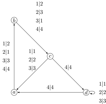
FIGURE IV.5 – Un contre-exemple connexe à la conjecture de [65], construit en prenant deux automates cycliques sur des alphabets disjoint puis en identifiant certains états. Le groupe engendré est d'ordre 8503056 = 2^4 3^{12} > 25 \times 4!^4 .
