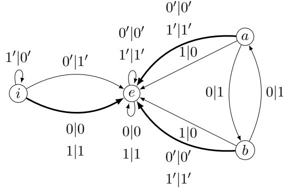
FIGURE I.20 – Produit direct puisé de la machine à additionner et de l’automate de la Basilique. Les nouvelles transitions sont en gras.
