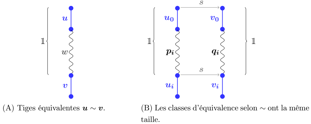
FIGURE II.9 – Equivalence \sim sur l'ensemble des tiges d'un arbre de la jungle.
