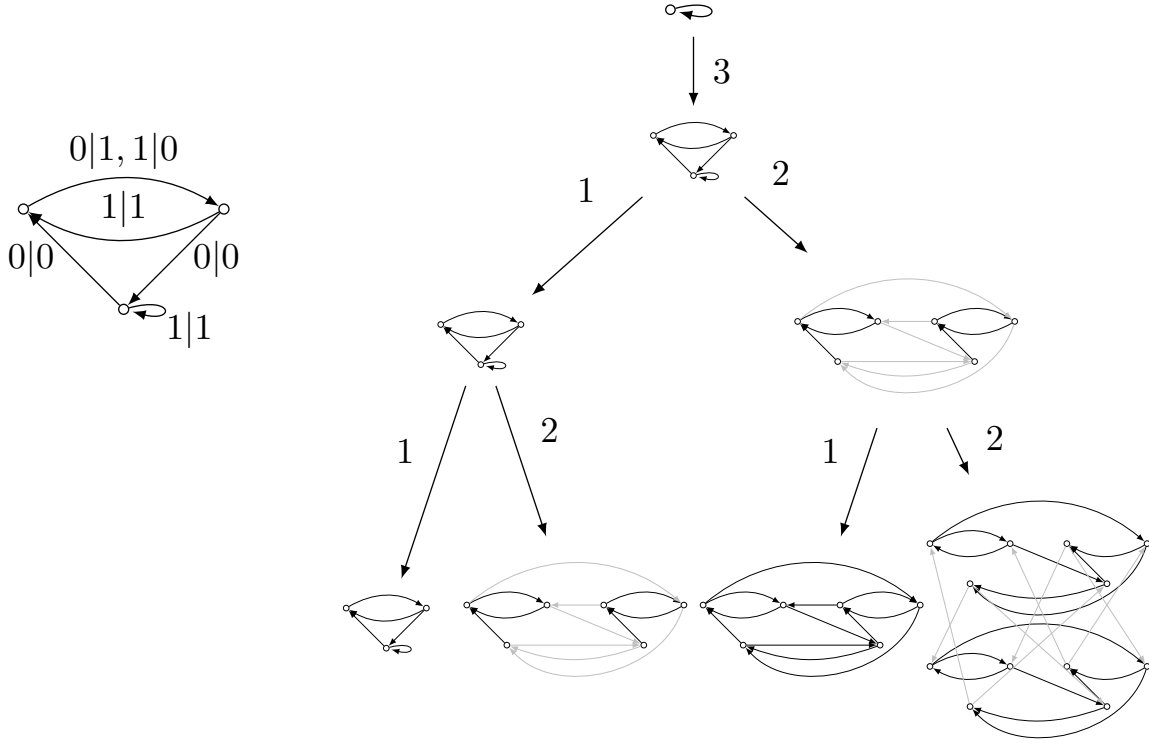
FIGURE II.2 – L'automate \mathcal{B} de Bellaterra et les 4 premiers niveaux de l'arbre lexicographique de Schreier \mathfrak{t}(\mathcal{B}) .
