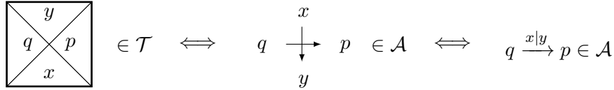
FIGURE III.11 – Le jeu de tuiles \mathcal{T}(\mathcal{A}) associé à l'automate \mathcal{A} .
