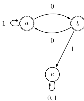
FIGURE III.6 – Un automate de Büchi dont le langage a pour entropie le logarithme du nombre d'or.
