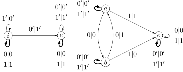
FIGURE I.18 – Produit direct bouclé de la machine à additionner et de l’automate de la Basilique. Les nouvelles transitions sont en gras.
