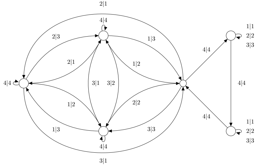
FIGURE II.11 – Un exemple d'automate avec un nombre d'états non-premier, pour lequel un analogue du théorème 3.22 peut être appliqué.
