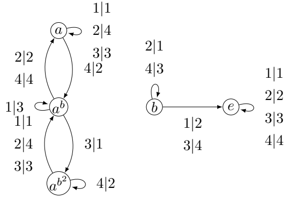
FIGURE I.24 – L'automate de Mealy \mathcal{H} engendrant le groupe d'Heisenberg H_3(\mathbb{Z}) .
