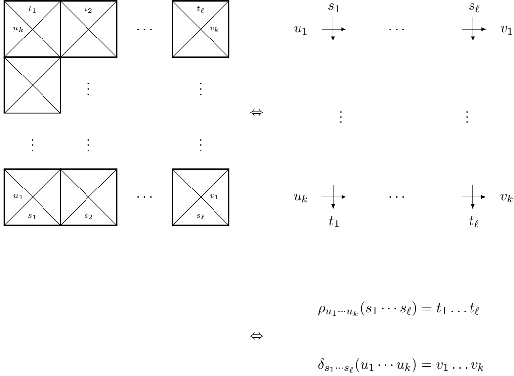
FIGURE III.12 – Correspondance entre pavages partiels, diagrammes en croix et actions de l'automate.
