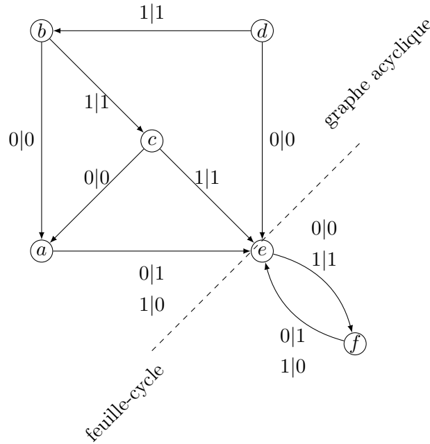
FIGURE IV.2 – Un automate avec cycles sans échappatoire, engendrant un groupe d'ordre 256.
