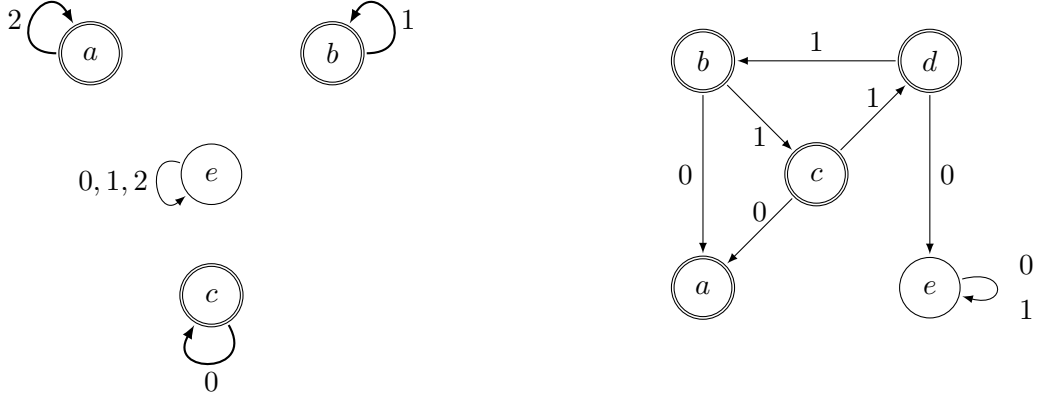
FIGURE III.4 – Les automates stables de l'automate des tours de Hanoi \mathcal{B}(H^{(3)}) (à gauche) et de l'automate de Grigorchuk (à droite).
