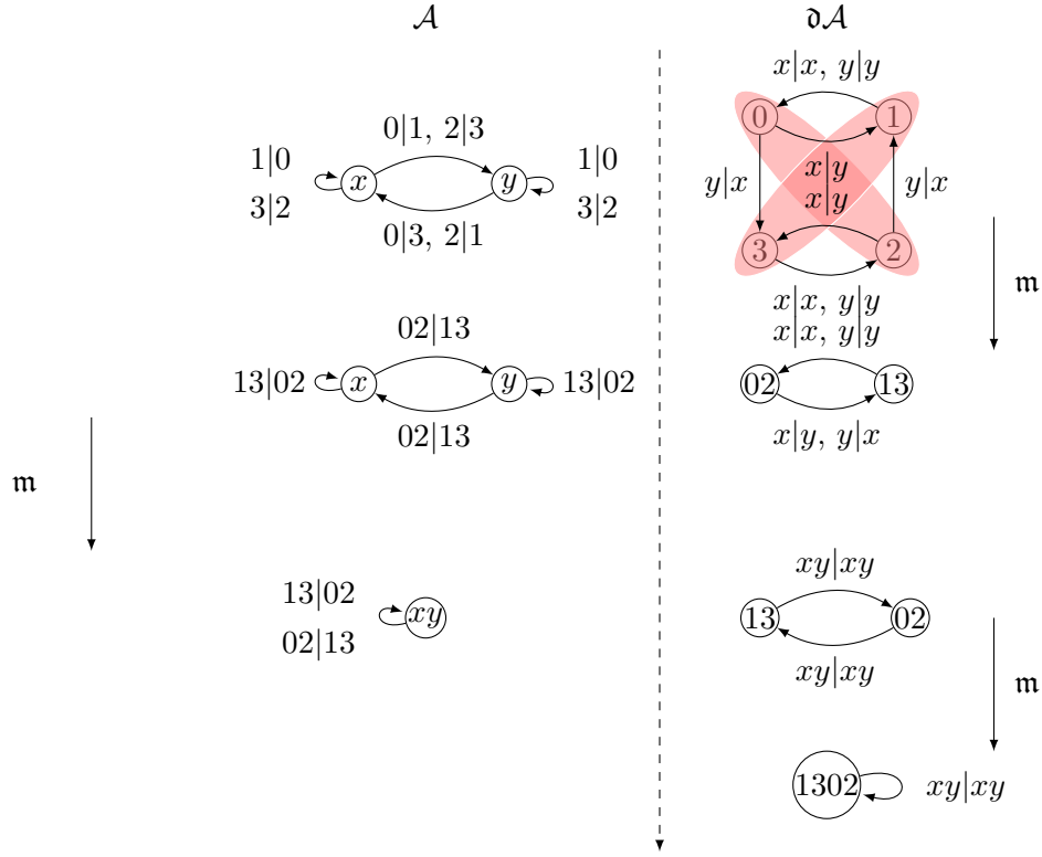
FIGURE I.21 – Une suite de m\delta -réductions conduisant à un automate trivial.
