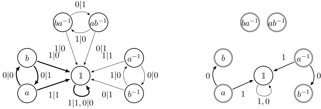
FIGURE III.2 – Le noyau (à gauche) et l'automate stable (à droite), associés à l'automate de la Basilic (figure I.17, arêtes du noyau en gras ).
