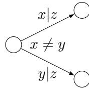
FIGURE I.2 – Configuration interdite pour les automates inversibles.
