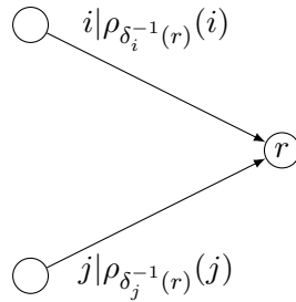
FIGURE II.5 – Dans un automate biréversible, pour tout état r et toutes lettres i \neq j , \rho_{\delta_i^{-1}(r)}(i) \neq \rho_{\delta_j^{-1}(r)}(j) .
