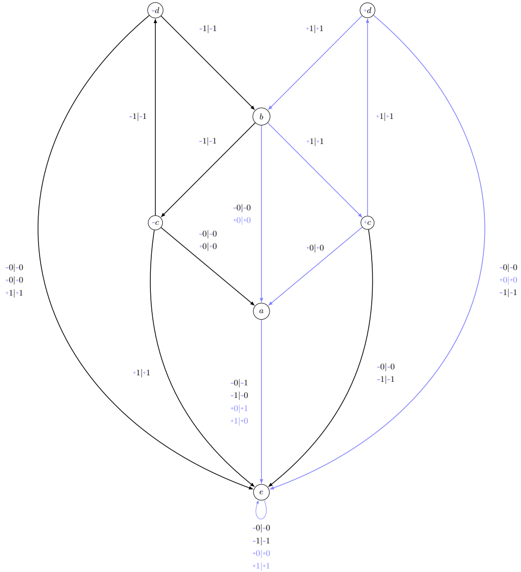
FIGURE I.1 – Ceci est un automate de Mealy.
