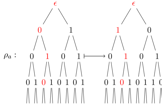
FIGURE I.4 – Action de l'état a de l'automate de Grigorchuk sur l'arbre binaire.
