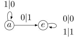
FIGURE I.7 – La machine à additionner, engendrant le groupe \mathbb{Z} .
