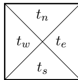
FIGURE III.10 – Une tuile de Wang.
