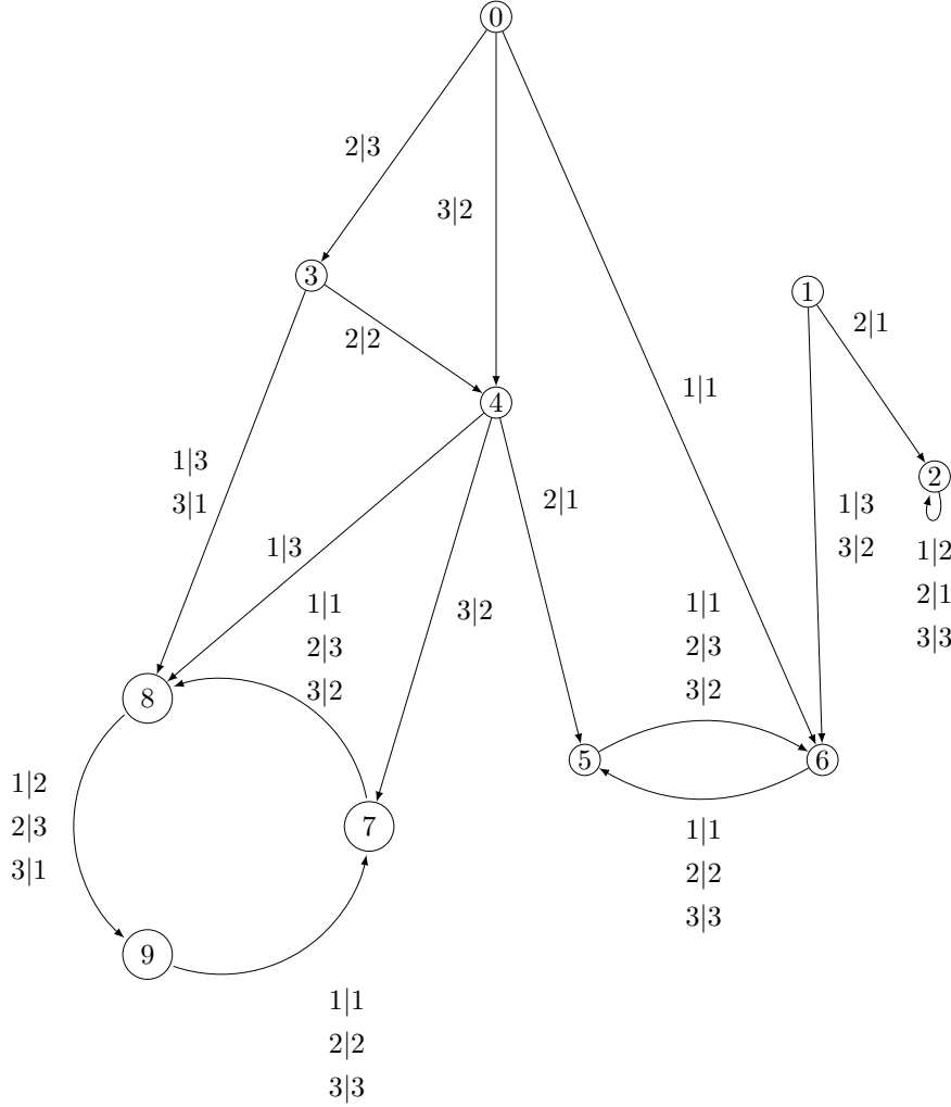
FIGURE I.12 – Un automate à cycles sans échappatoire à 10 états et 3 lettres.
