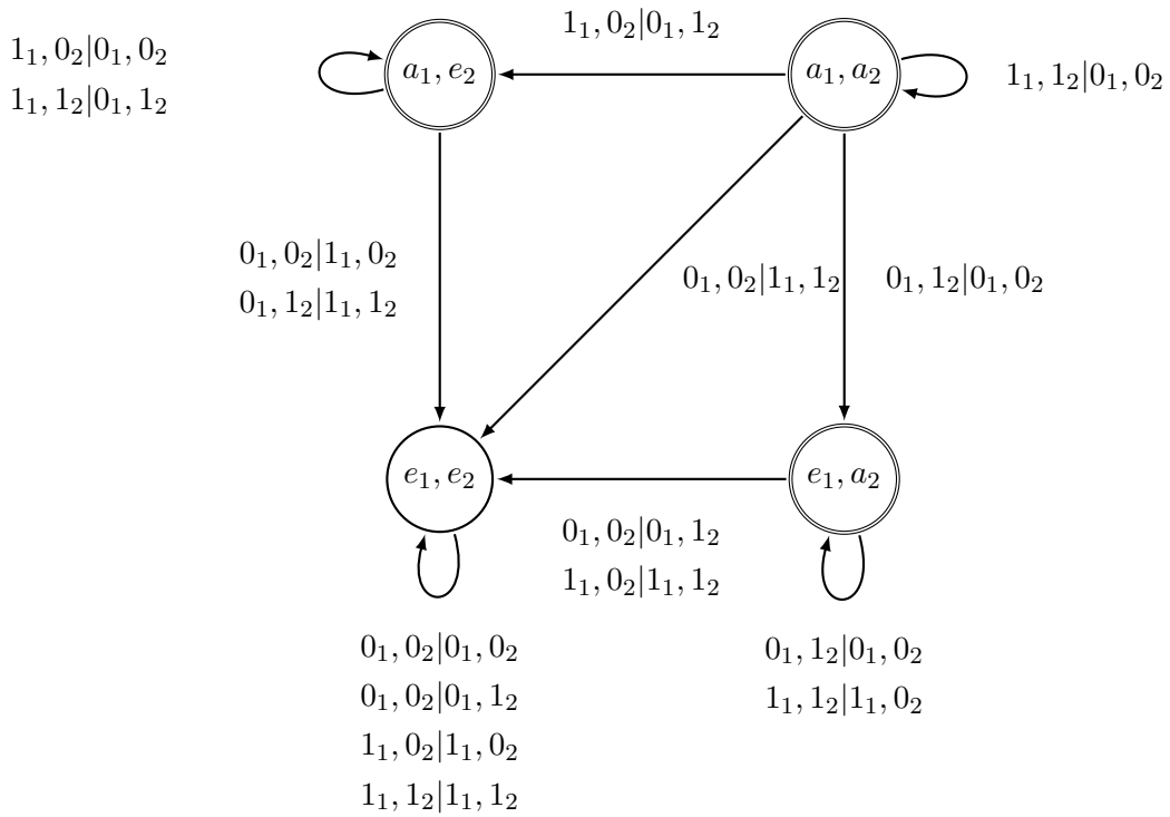
FIGURE III.7 – Construction de Cain pour \mathbb{Z}^2 .
