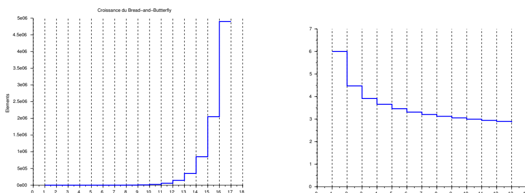
FIGURE I.5 – Croissance \gamma(\ell) du groupe engendré par le Bread-and-Butterfly (à gauche), et fonction \ell \mapsto \sqrt[\ell]{\gamma(\ell)} (à droite)
