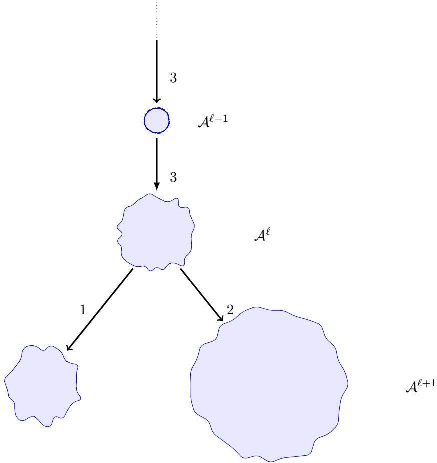
FIGURE II.4 – Un automate connexe, inversible, réversible et non-coreversible à trois états agit transitivement par niveau, sinon on trouverai un 1 dans l'arbre de Schreier.
