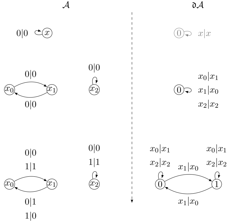
FIGURE IV.6 – Un exemple de \epsilon\mathfrak{d} -extension. On commence par l'expansion selon (0, 1)(3) puis dans le dual on effectue l'expansion \epsilon_{(0,1)}
