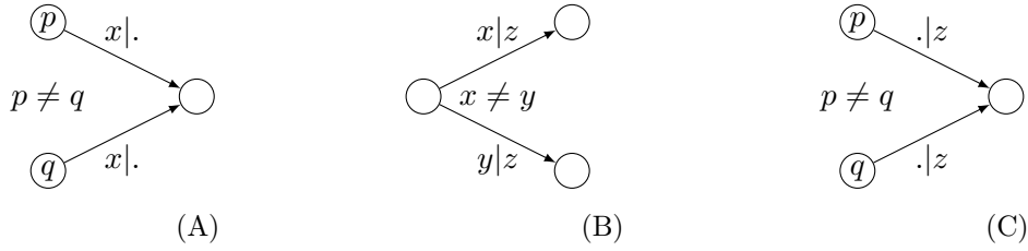
FIGURE I.10 – La configuration (A) est proscrite pour les automates réversibles, la configuration (B) l'est pour les inversibles, et la configuration (C) pour les coréversibles.
