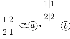
FIGURE I.6 – Un automate de Mealy inversible mais pas réversible, engendrant K_4 = \mathbb{Z}/2\mathbb{Z} \times \mathbb{Z}/2\mathbb{Z} .
