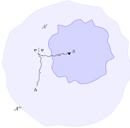
FIGURE I.15 – Principe d'un automate fractal : quitte à se placer dans une puissance supérieure, on peut arriver dans n'importe quel élément après avoir stabilisé un préfixe quelconque.
