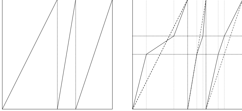
FIGURE 8. Une source sans mémoire, une chaîne de Markov.
