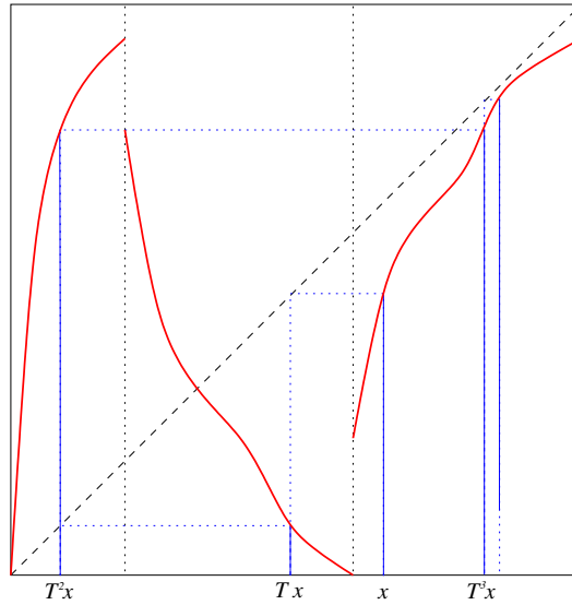
FIGURE 3. Une orbite créée par une source dynamique et le mot émis associé cbac...
