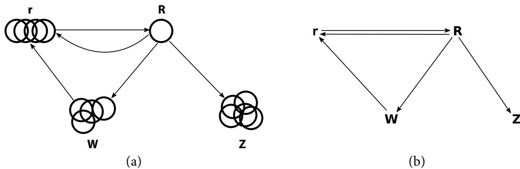
Figure 3.3 – Structures de données de l'ordonnanceur (a) et transitions des processus (b).
