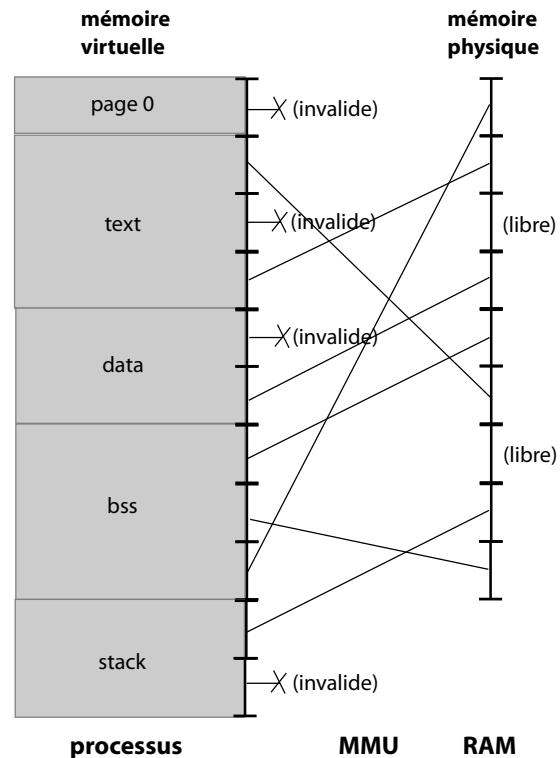
Figure 3.6 – Mémoire virtuelle d'un processus. (Les pages invalides des sections text et data seront chargées de manière paresseuse.)
