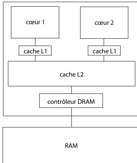
Figure 3.9 – Le processeur et ses caches
