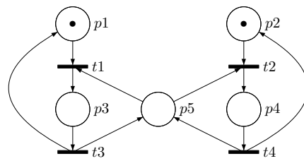
FIGURE 1 – Un réseau de Petri représentant deux processus en exclusion mutuelle
